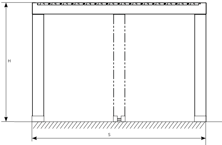
Yandan Görünüş / Side View
